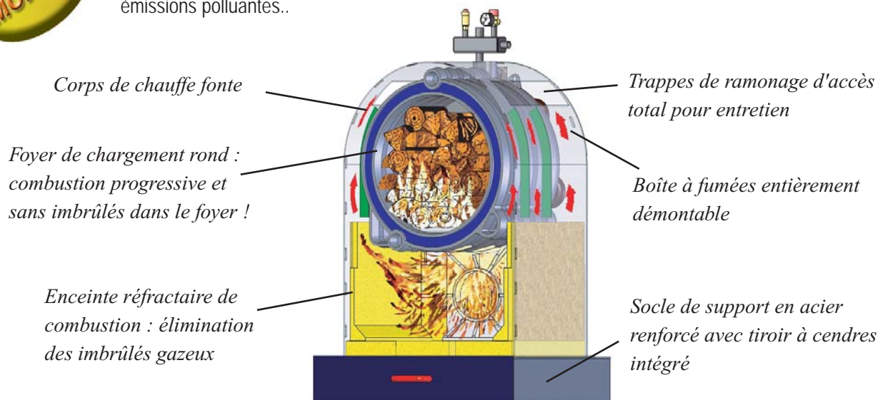
Corps de chauffe nu
