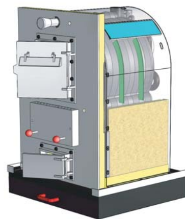
Corps de chauffe avec façade
